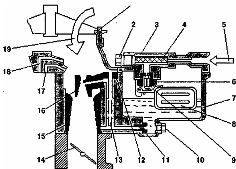
Рис. 6. Схема главной дозирующей системы карбюратора К-126: 1 - входной воздушный патрубок; 2 - пробка топливного фильтра; 3 - крышка поплавковой камеры; 4 - топливный фильтр; 5 - вход топлива от бензонасоса; 6 - клапан поплавковой камеры; 7 - корпус поплавковой камеры; 8 - поплавок; 9 - игла клапана поплавковой камеры; 10 - пробка главного топливного жиклера; 11 - главный топливный жиклер; 12 - главный воздушный жиклер; 13 - эмульсионная трубка; 14 - дроссельная заслонка; 15 - большой диффузор; 16 - малый диффузор; 17 - распылитель экономайзера; 18 - распылитель ускорительного насоса; 19 - вход воздуха
